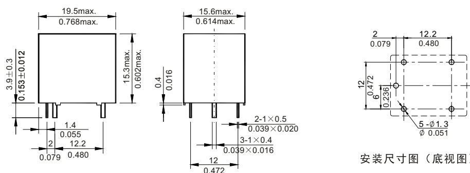
外形尺寸图
